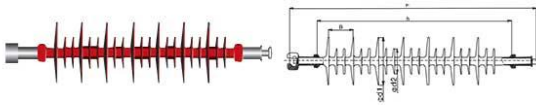
69kV(66kV、63kV) 棒形悬式复合绝缘子示意图 69kV(66kV、63kV) Composite Long Rod Suspension Type Insulator Schematic Diagram
